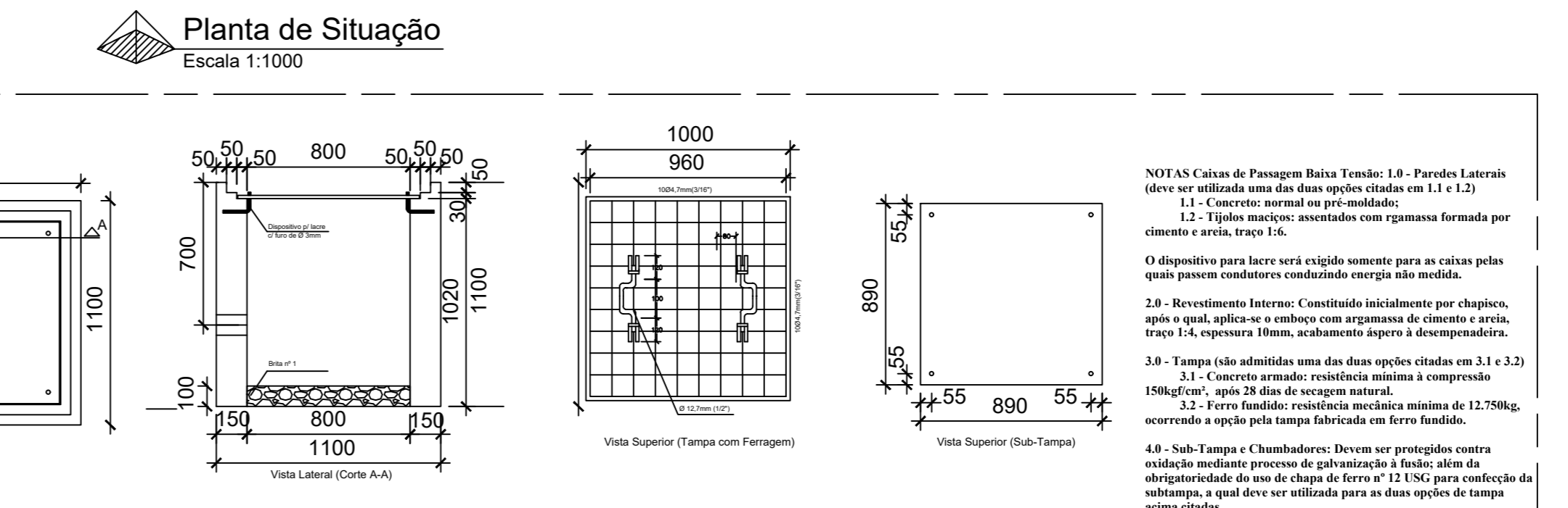
Caixa de passagem - Padrão Equatorial Sem escala
