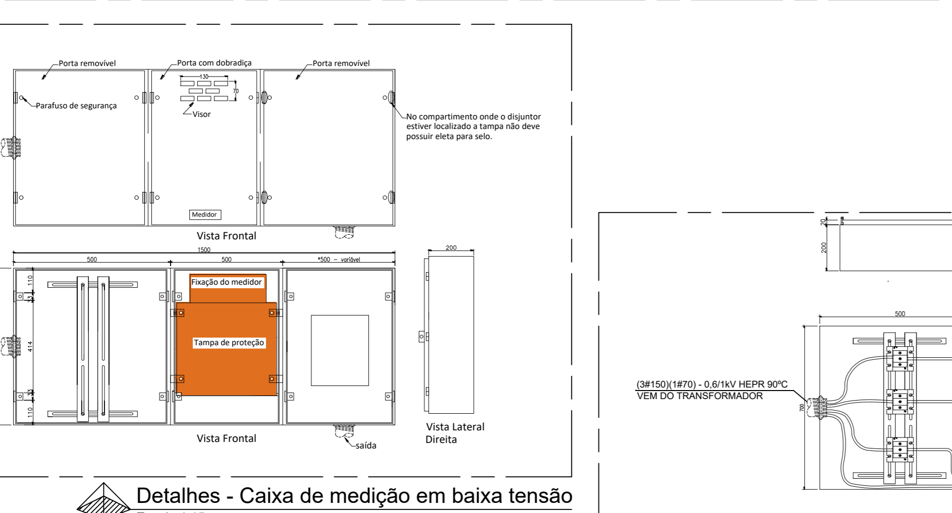
Detalhes - Caixa de medição em baixa tensão Escala 1:15
