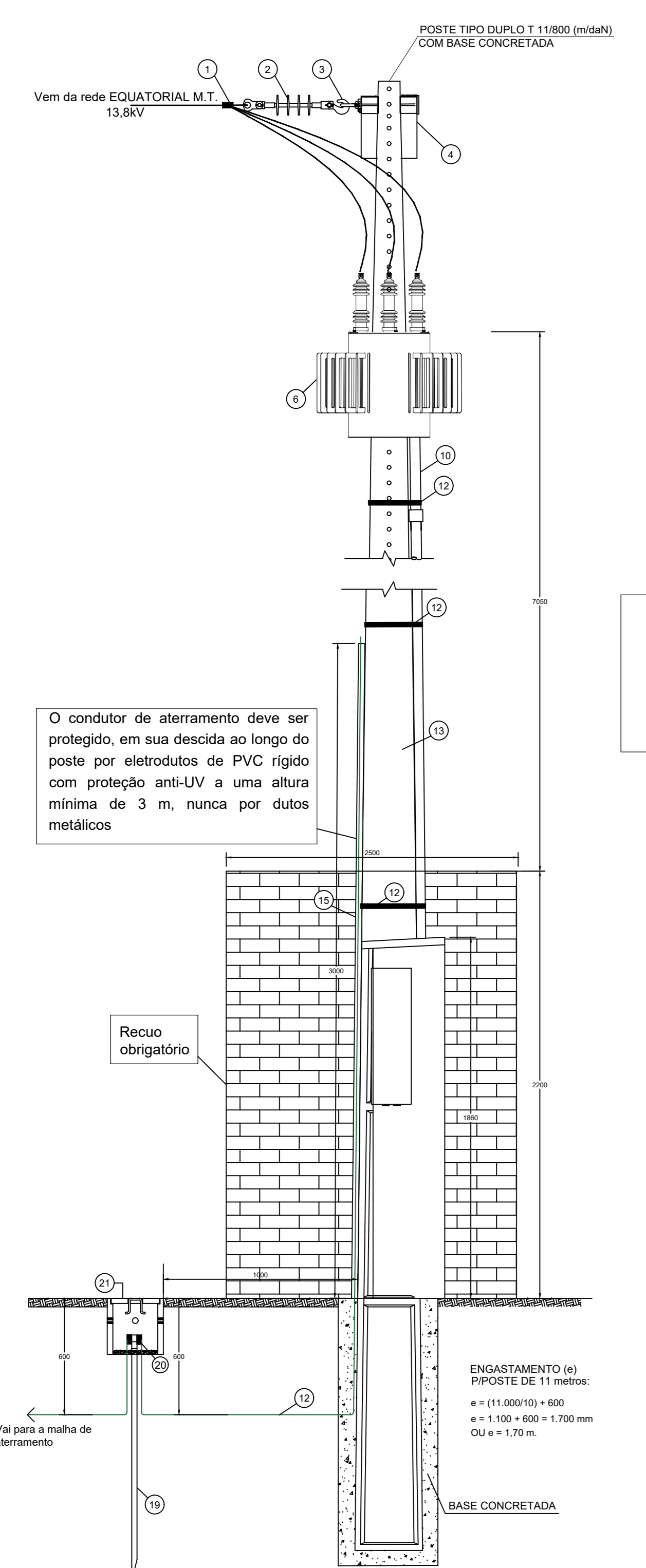
Corte B-B Escala: 1:20
