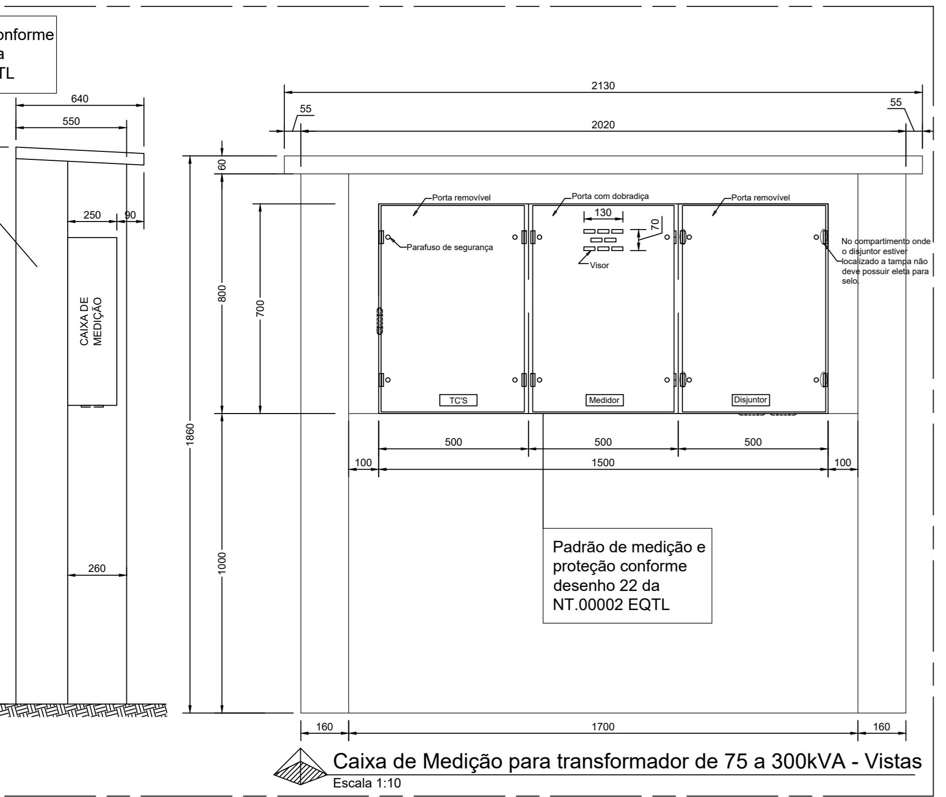
Caixa de Medição para transformador de 75 a 300kVA - Vistas Escala 1:10
