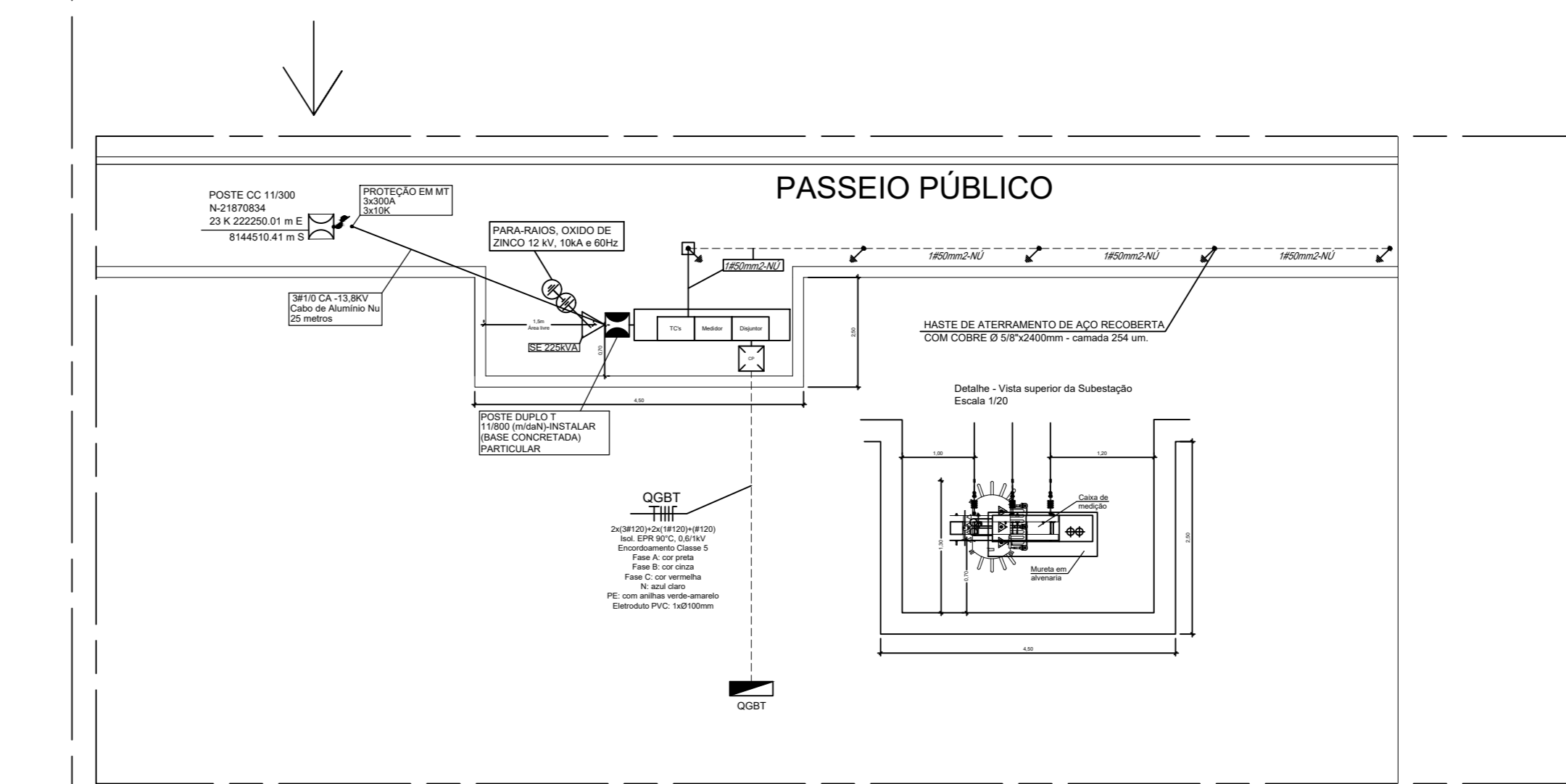
Planta Baixa - Implantação SEE 225kVA Escala 1:150
