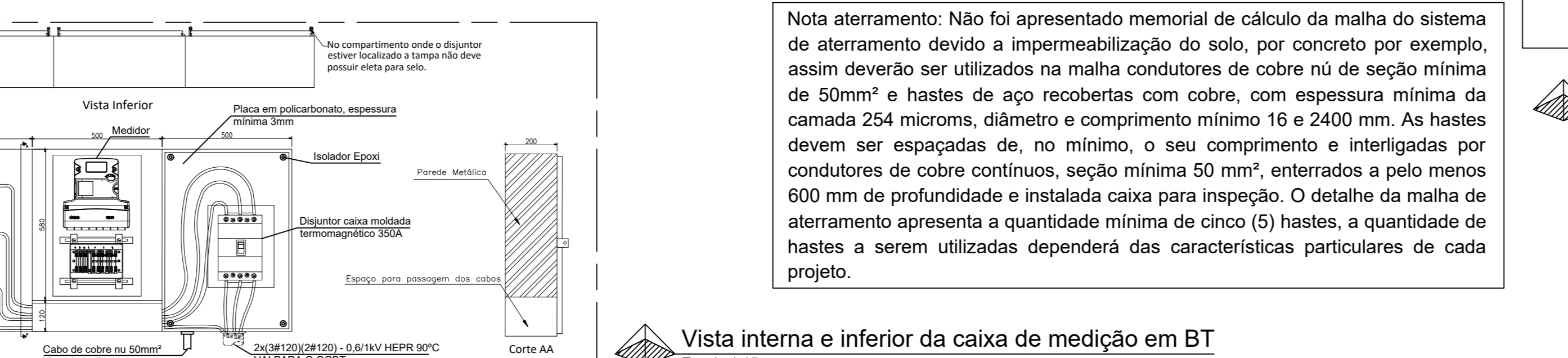
Vista interna e inferior da caixa de medição em BT Escala 1:15
